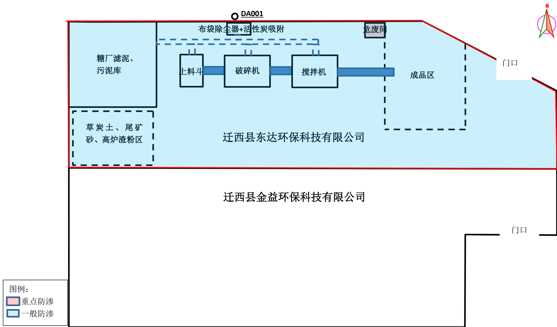
附图 3-3 项目生产车间防渗分区图 比例尺 1:500
