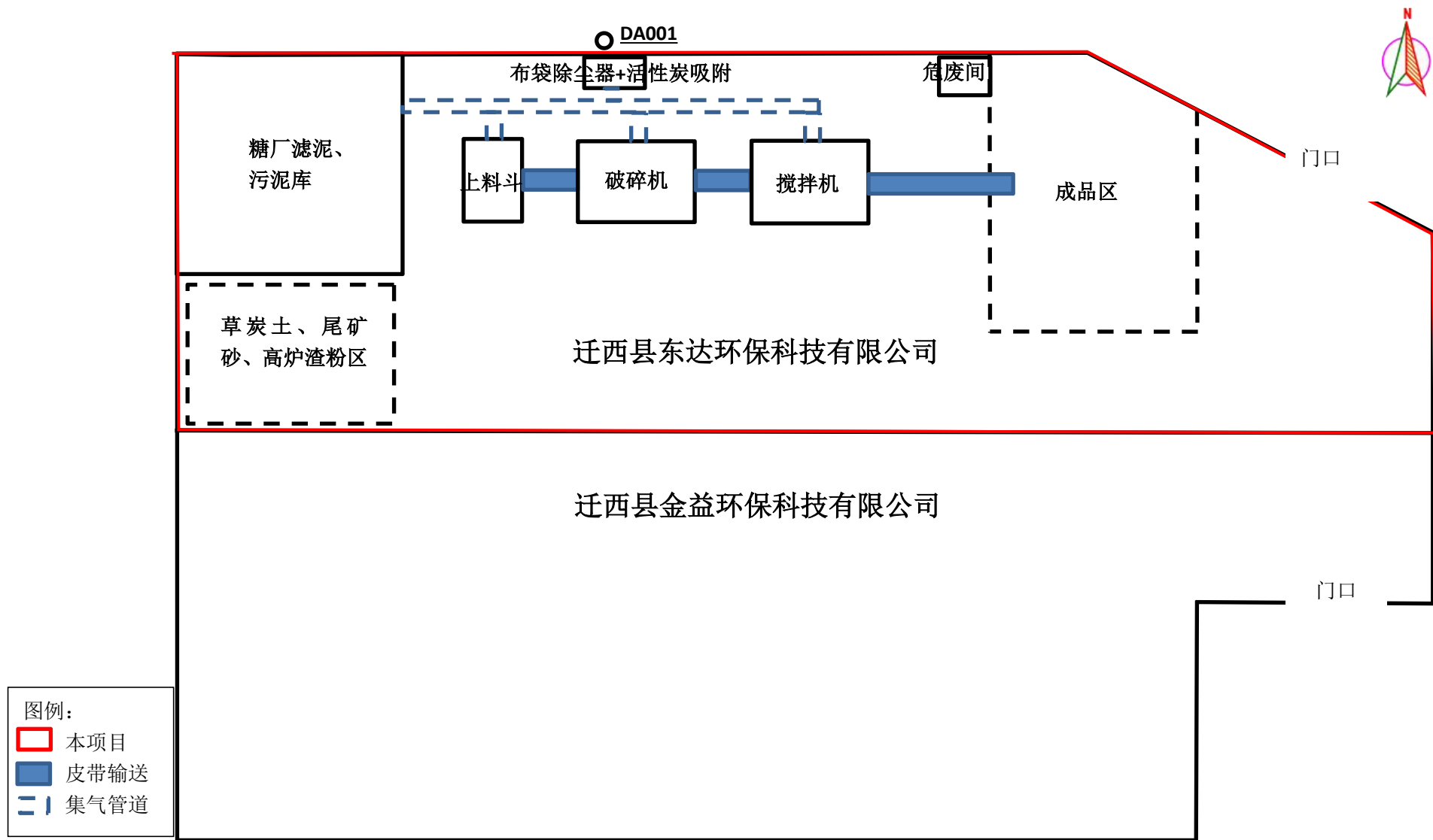
附图 3-2 项目生产车间平面布置图 比例尺 1:500
